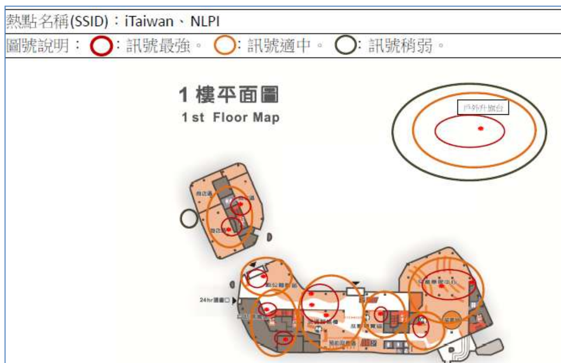
圖 82 本館無線網路上網熱點標示圖
