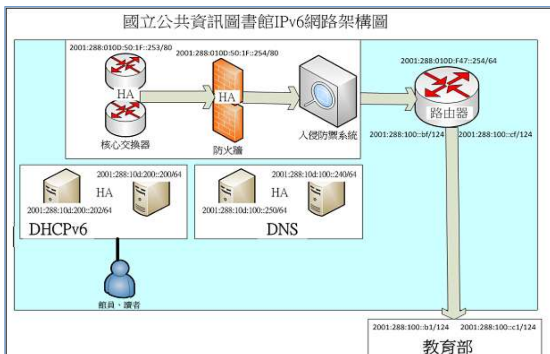
圖 81 本館 IPV6 網路架構圖
