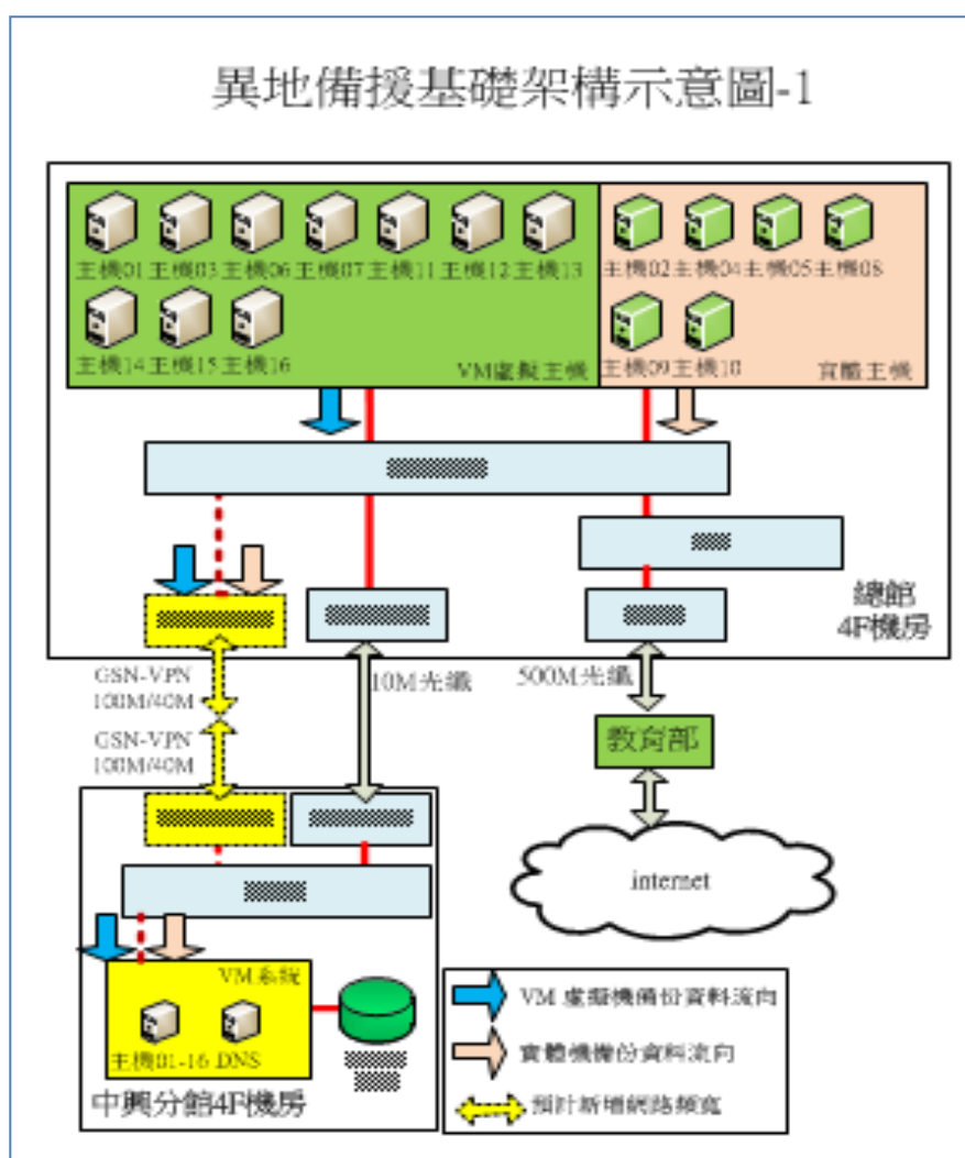
圖 83 異地備援基礎架構示意圖
