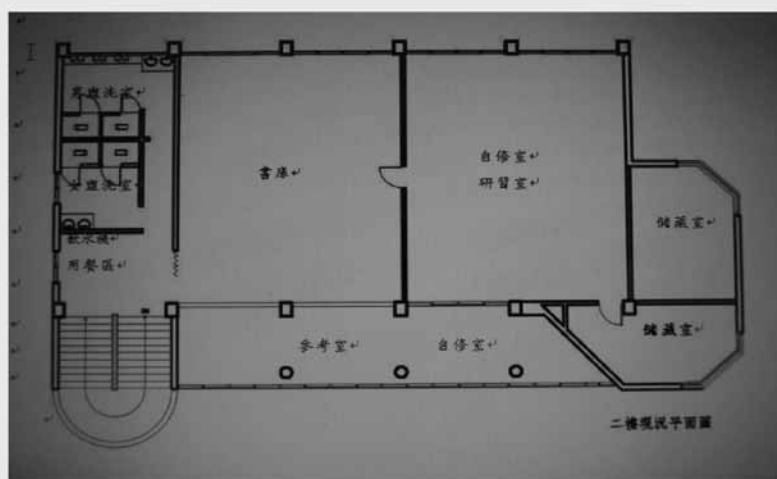
土庫鎮立圖書館二層現況平面圖
