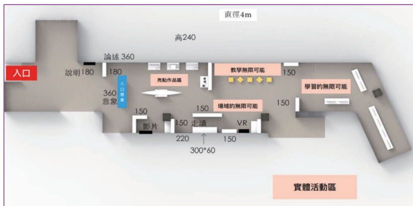
圖3 平配圖
