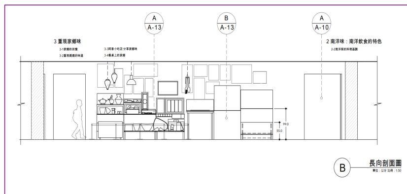
圖6 剖面圖
