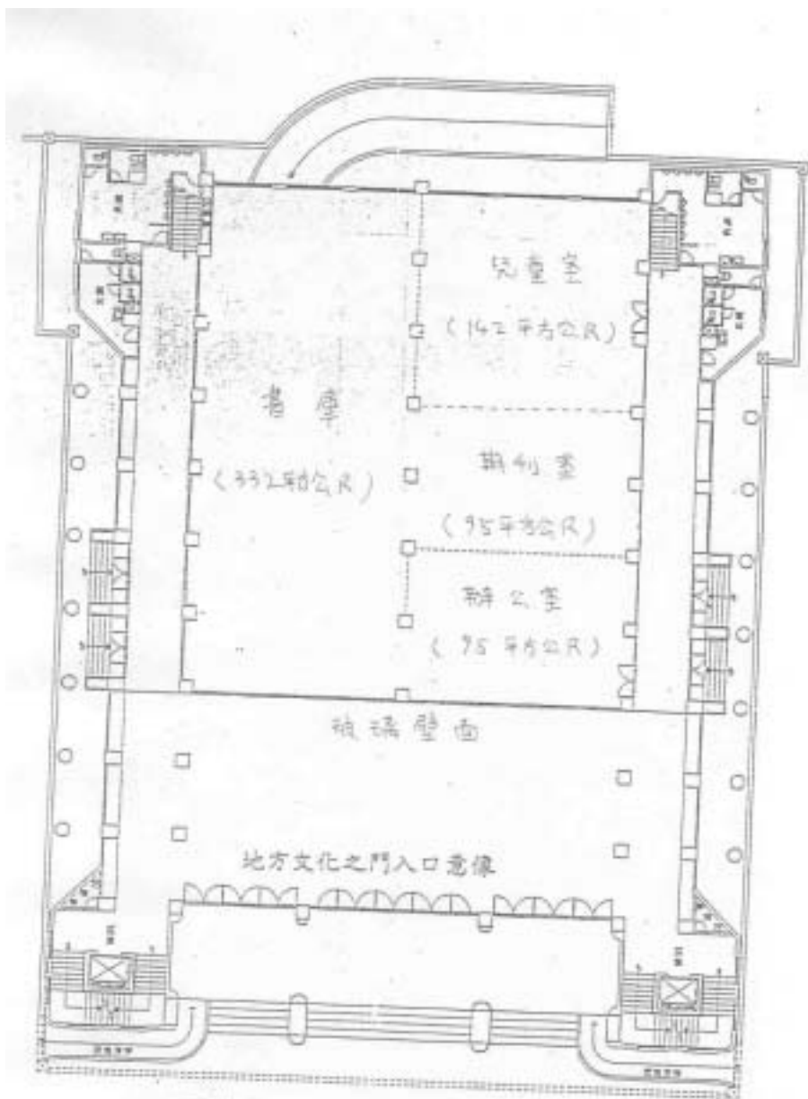
以文圖書館館舍再造一樓平面配置圖
