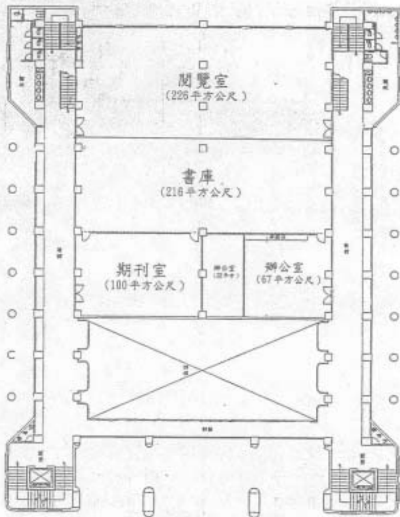
以文圖書館二樓平面圖 (2002/05)
