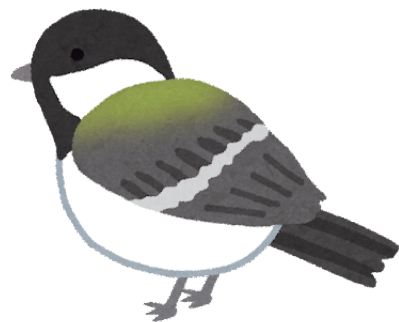
大山雀
