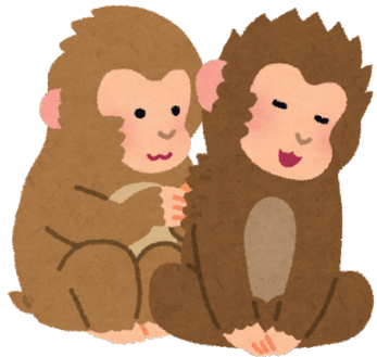
日本獼猴
